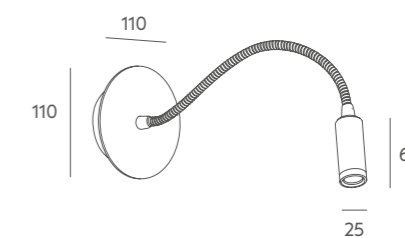
Flexible arm / Brazo flexible 380
